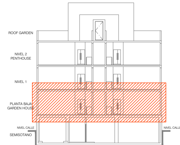
CORTE ESQUEMATICO
